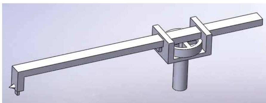
Εικ. 7. Άνω: Ανάπτυγμα της αναπαράστασης του μηχανισμού κίνησης του δείκτη. Μέσον: Τομή του μηχανισμού του δείκτη (αριστερά) και κοιτινή άποψη του εξαρτήματος καλύμματος κεφαλής (δεξιά). Κάτω: Αναπαράσταση του συναρμολογημένου μηχανισμού του δείκτη (από διδακτορική διατριβή Αναστασίου Μ.22).
