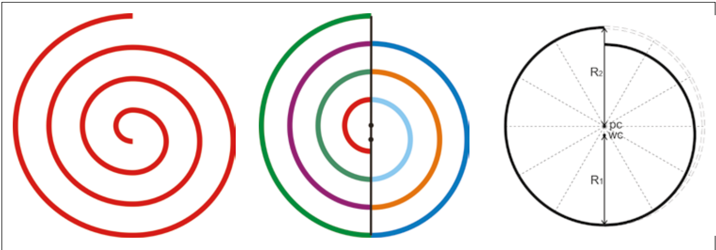
Εικ.8. Αριστερά: Η Αρχιμήδεια σπείρα (Τάξη-Α). Κέντρο: Η Σπείρα με Δύο Κέντρα (Τάξη- C). Δεξιά: Το πρόβλημα της εκκεντρότητας στις σπείρες της Τάξης-C του Μηχανισμού των Αντικυθέρων απεικονίζεται στο δεξιό ημικύκλιο.
