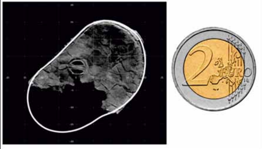
Εικ. 9. Άνω: Η καμπύλη που περιγράφεται από την οδηγητική καμπύλη του Θραύσματος D, προσομοιώνει την Εξίσωση του Χρόνου όπως υπολογίζεται για την εποχή του Πτολεμαίου. Κάτω αριστερά: Η οδηγητική καμπύλη του θραύσματος D. Κάτω δεξιά: Σύγκριση με τον χάρτη που αποτυπώνεται στο νόμισμα των 2 ευρώ (παραχώρηση: Κ. Ευσταθίου).
