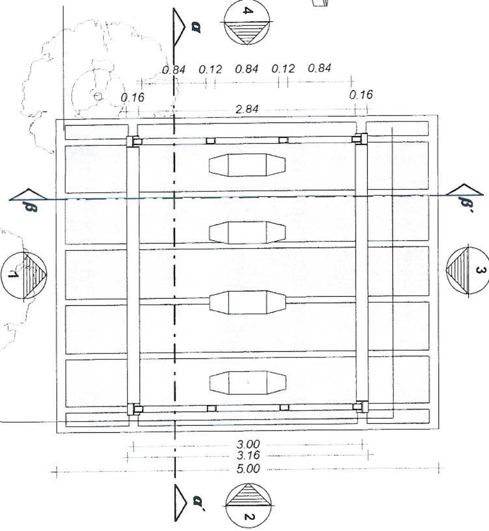
ΑΝΟΨΗ
