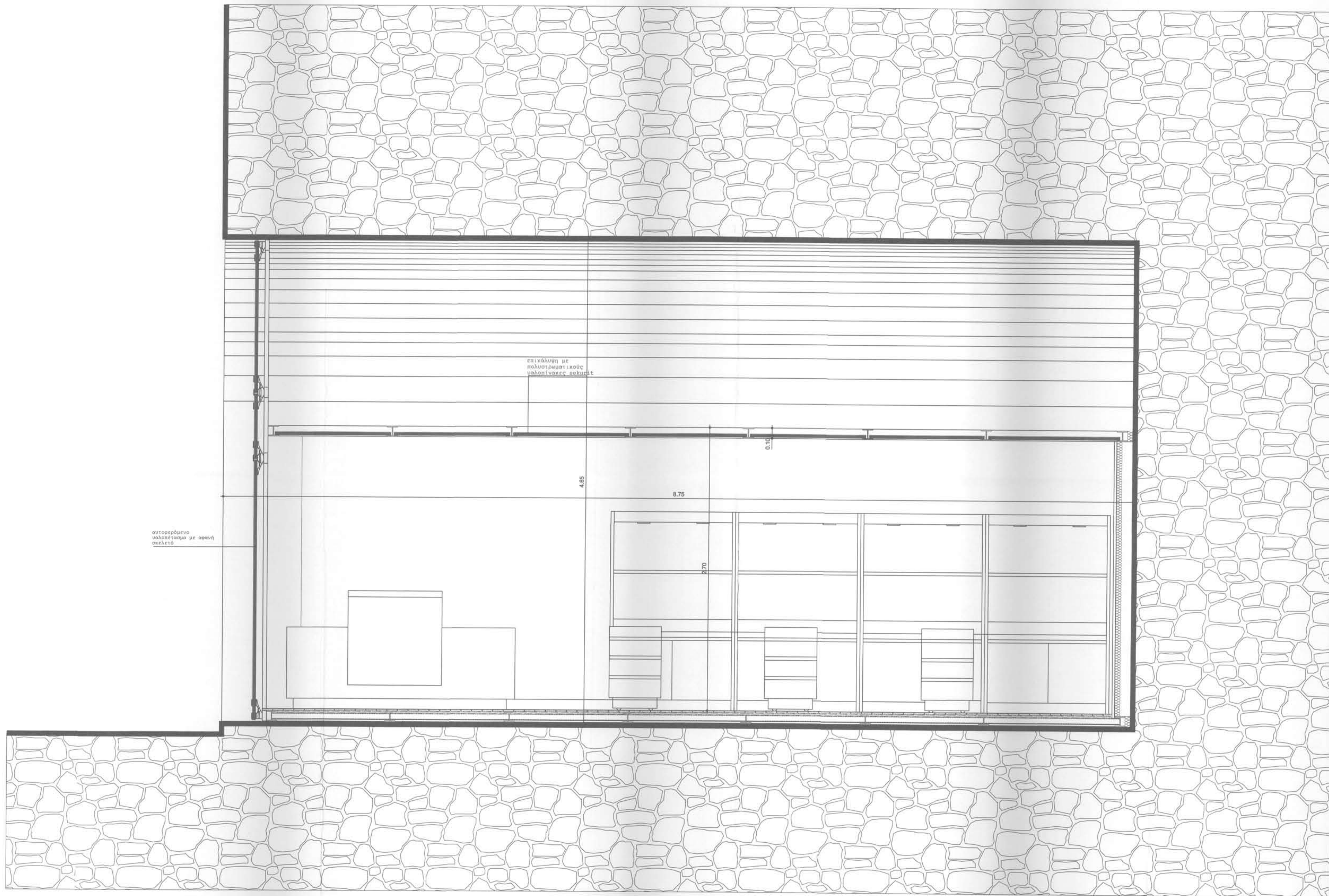
ΤΟΜΗ Β-Β
